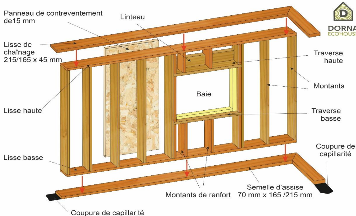
Éléments de l'ossature d'une partie de mur comportant une ouverture
